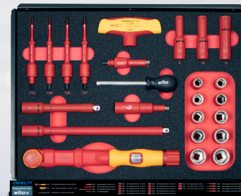
Tournevis dynamométrique TorqueVario®
